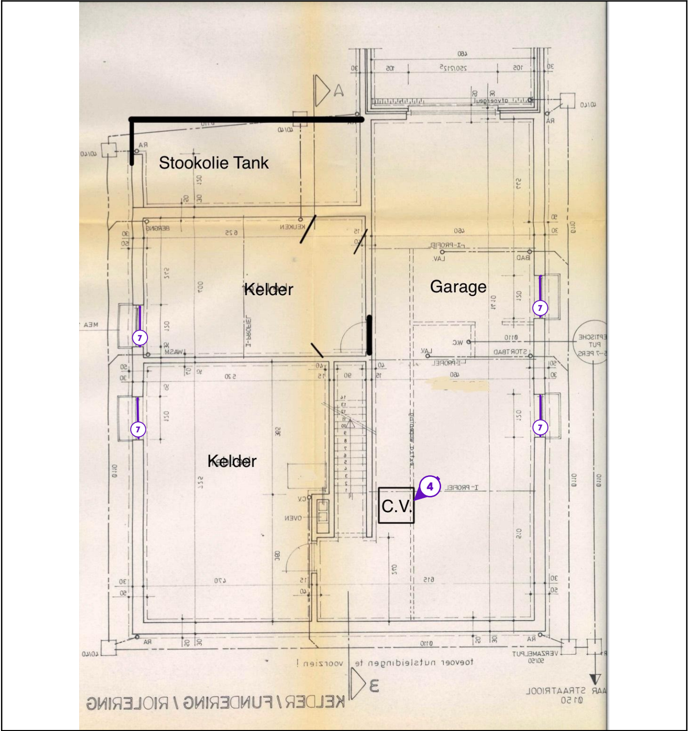
Legende van plan 1.1: Kelderverdieping
