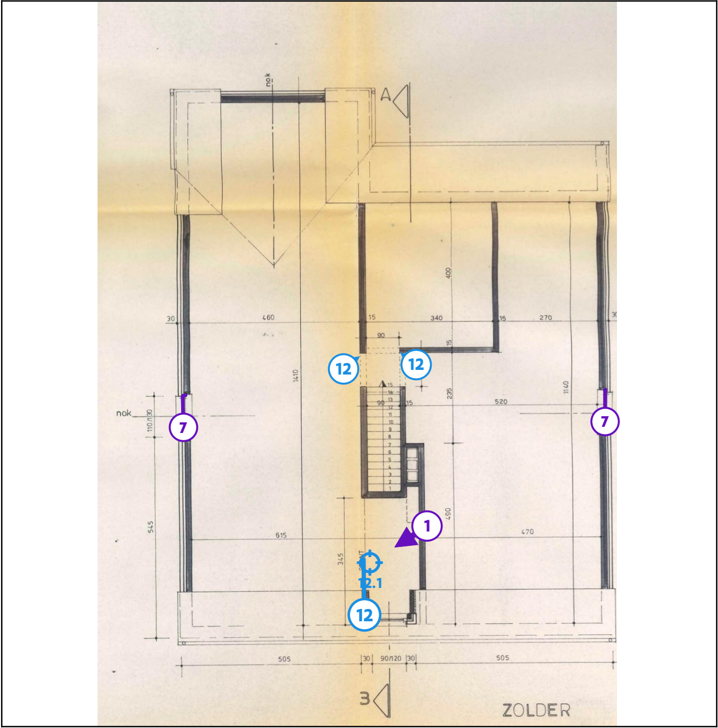
Legende van plan 1.4: Zolderverdieping
